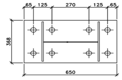
BASE PLATE D2A & D2B
