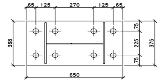
BASE PLATE D1
