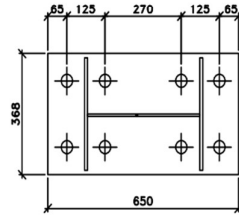
BASE PLATE D2A & D2B
