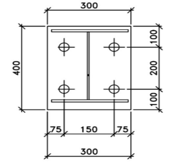
BASE PLATE D2
