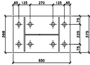
BASE PLATE D1
