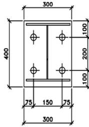
BASE PLATE D2
